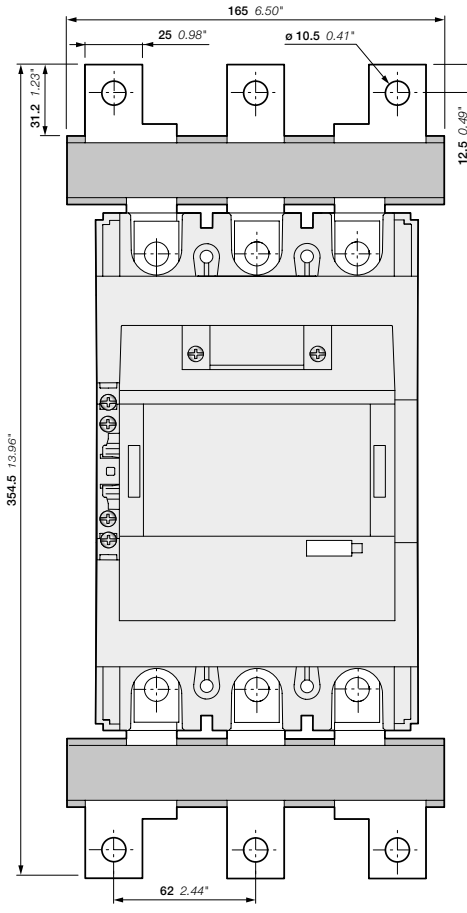
AF265, AF305, AF370-30-11 + LW370 terminal enlargement
