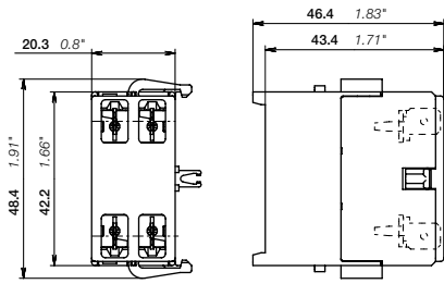
CA6-11E-F, CA6-11M-F, CA6-11N-F
