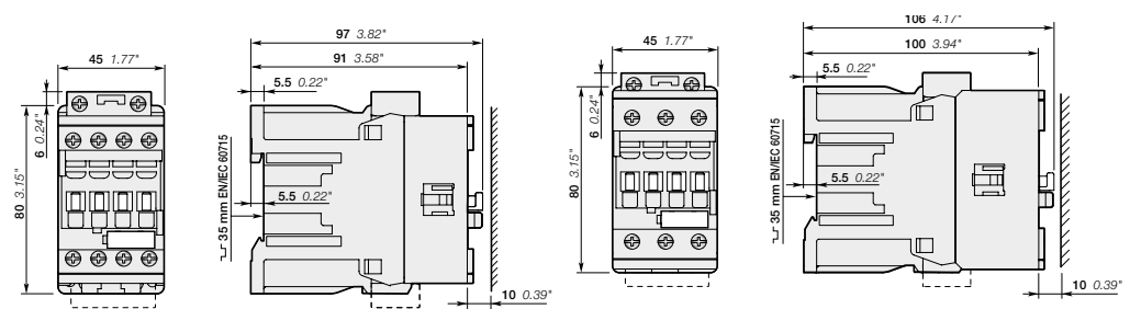
AF26Z, AF30Z, AF38Z
