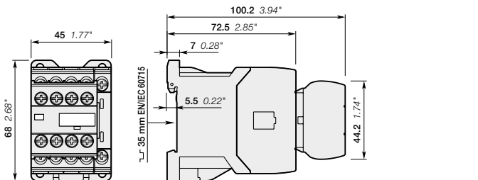
NSL44E, NSL53E, NSL62E, NSL71E, NSL80E
