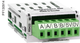
VW3A3620
