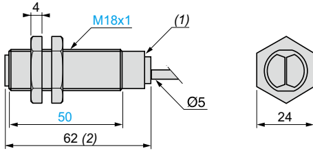
XU●N18●●341
